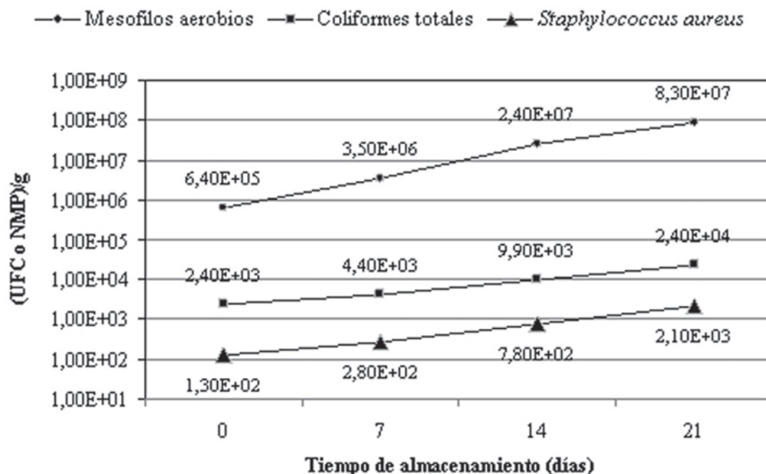
FIGURA 4. Comportamiento de las bacterias mesófilas aerobias, coliformes totales y Staphylococcus aureus en el queso blanco artesanal tipo telita durante 21 días de almacenamiento a \pm 5^\circ\text{C} .
