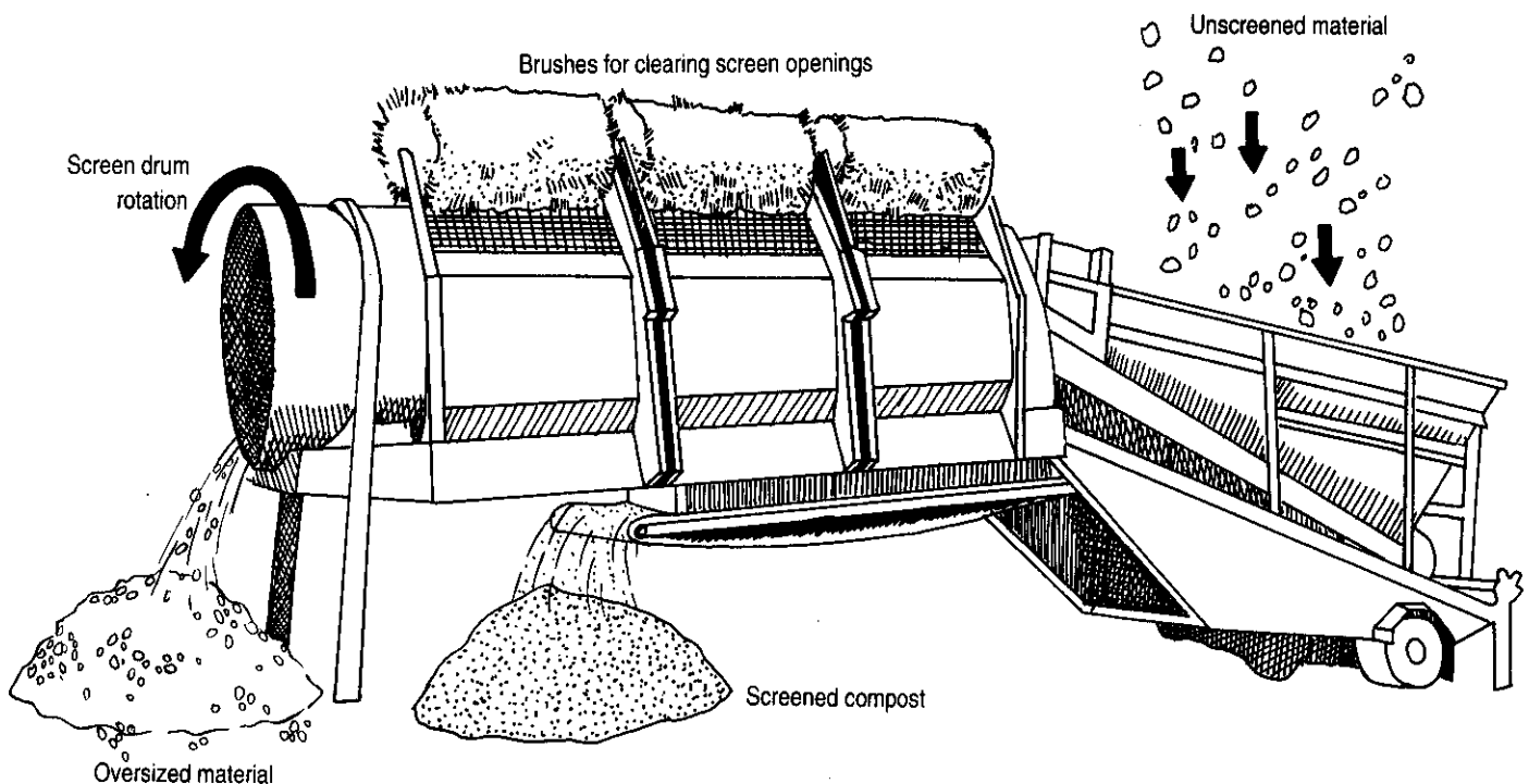
Figure 5.13 Trommel screen.
